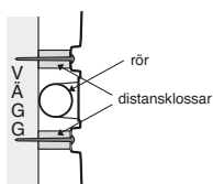
Fastsättning Alternativ B (uppifrån)
